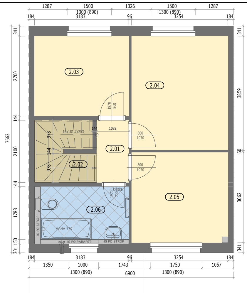
POZIČNÍ SCHÉMA - řada A
