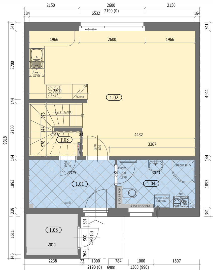
LEGENDA MÍSTNOSTÍ 1.NP – ŘADOVÝ DŮM R90
